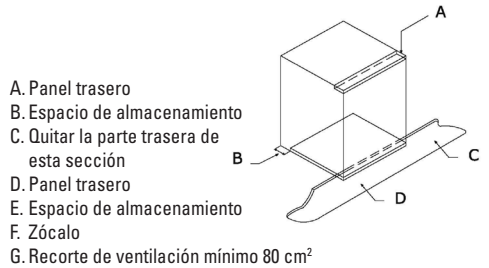
Fig. 8: Requisitos de ventilación y recorte para la instalación de un horno eléctrico simple en un armario alto.
