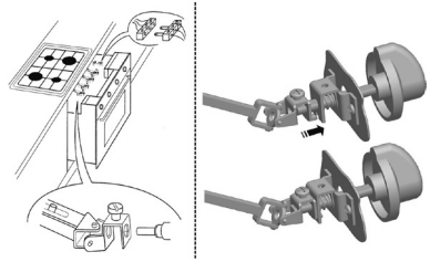
4. En caso de instalar hornos polivalentes, instalar los cardanes tal como se observa en la figura nº6.
